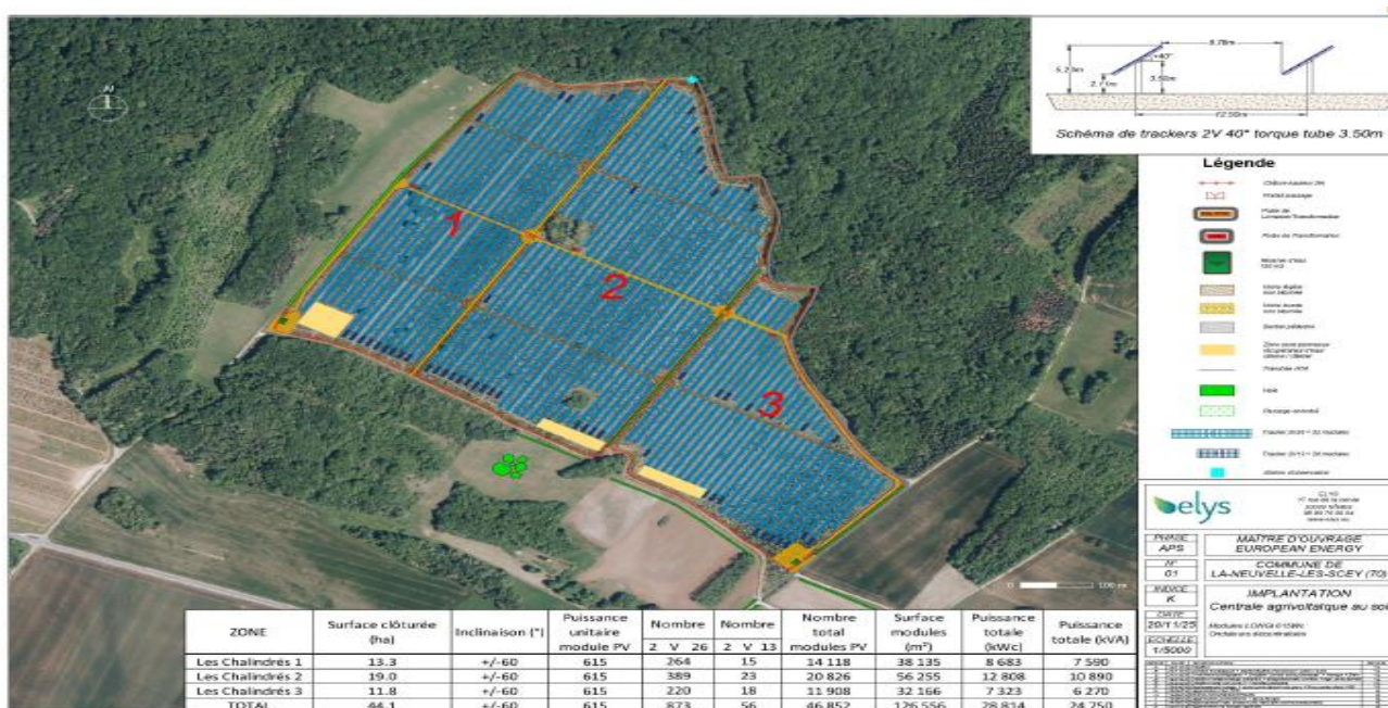
Figure 1: Schéma d'implantation du projet (source : étude d'impact)
